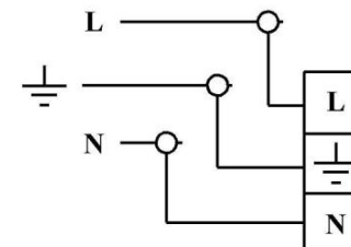
Рис1. Схема подключения светильника.
